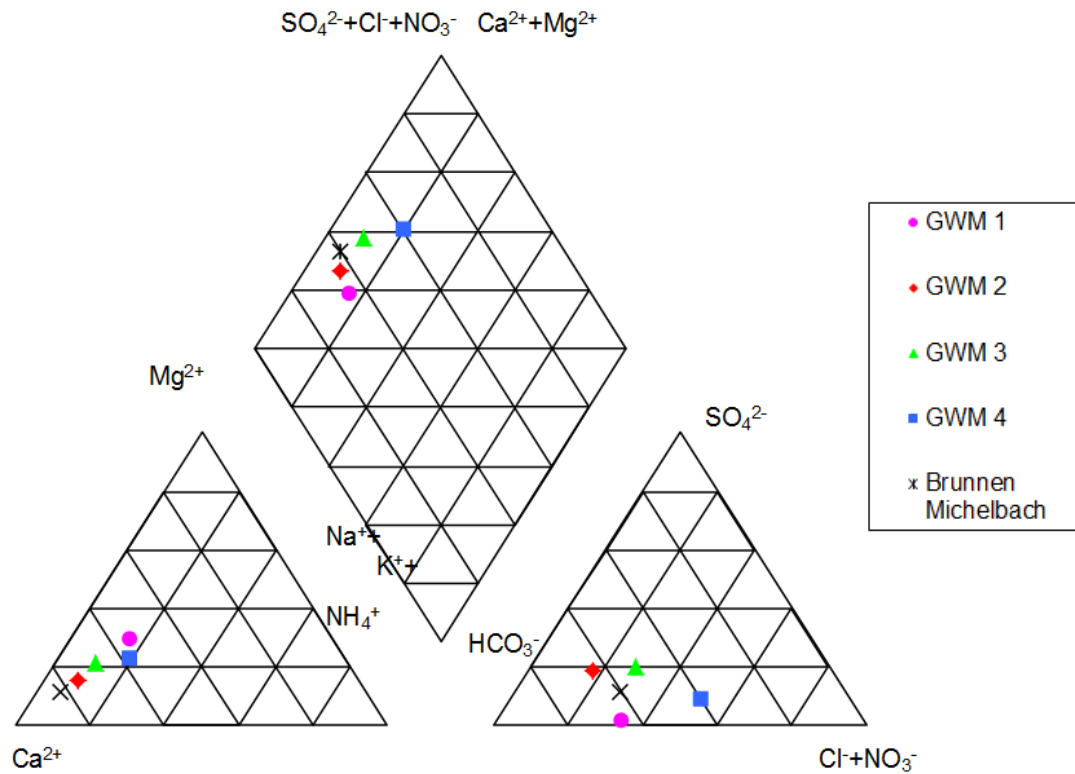
Abbildung 2: Darstellung der Ionenverhältnisse im Piper-Diagramm für den 19.03.2018 - Bereich ehemaliger Gemeindemüllplatz Michelbach
