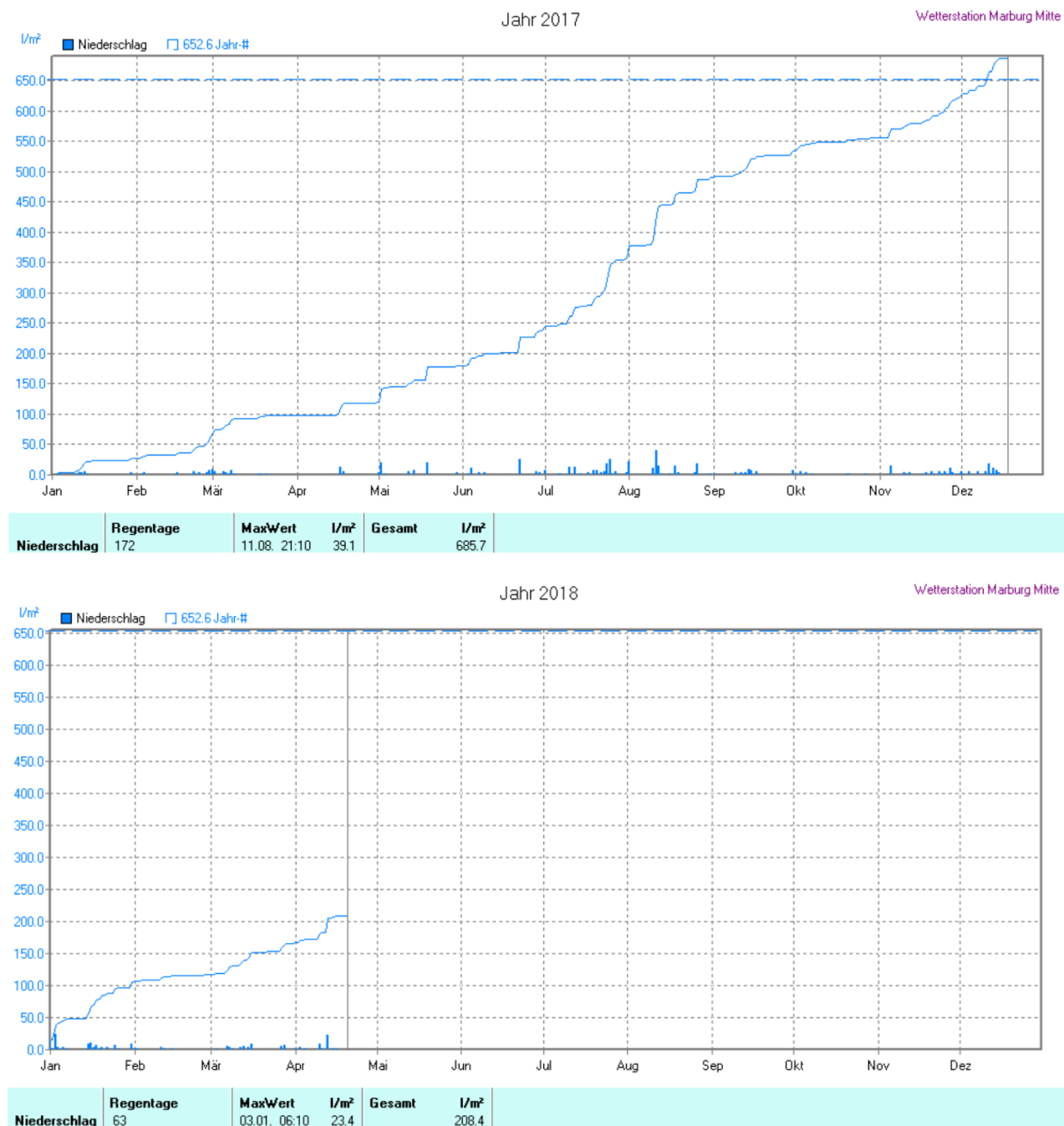
Abbildung 1: Jahresverläufe der Niederschläge 2017/2018 für die Wetterstation Marburg-Mitte (Stand 20.04.2018) (Quelle: www.wettereule.de )
