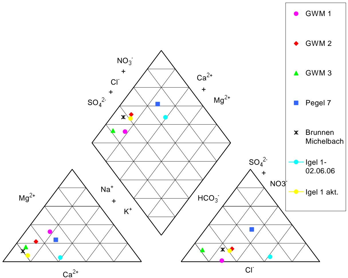
Abb. 1: Darstellung der Ionenverhältnisse im Piper-Diagramm für den 18.11.2008 sowie für die Erstbeprobung von GWM Igel 1 (02.06.2006).
