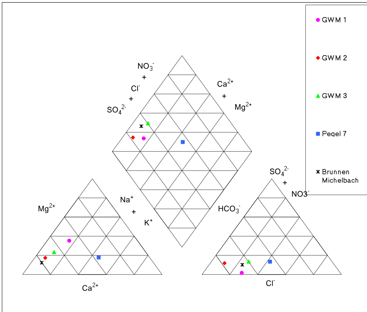
Abb. 1: Darstellung der Ionenverhältnisse im Piper-Diagramm für den 24.09.2012
