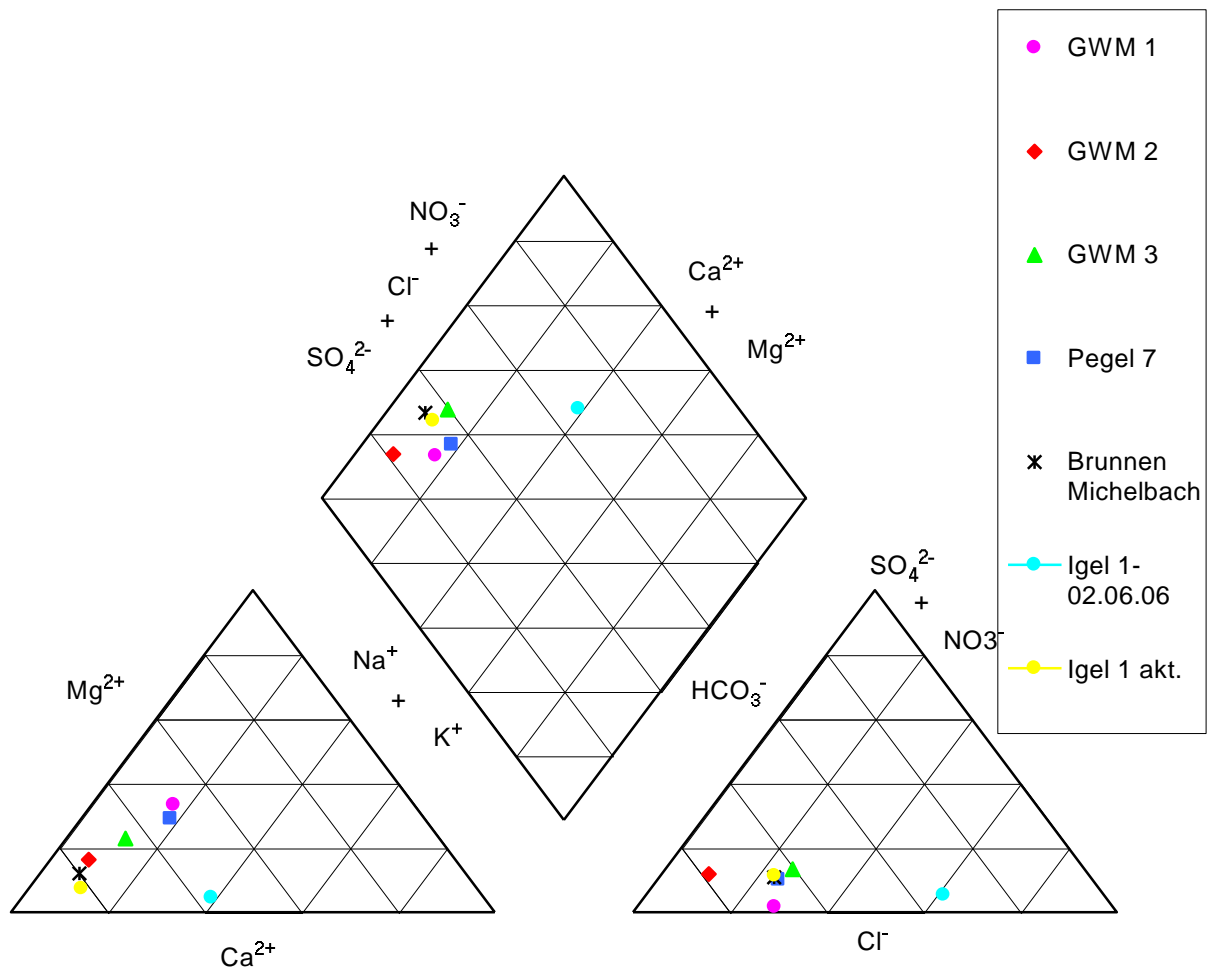
Abb. 1: Darstellung der Ionenverhältnisse im Piper-Diagramm für den 30.09.2009 sowie für die Erstbeprobung von GWM Igel 1 (02.06.2006).
